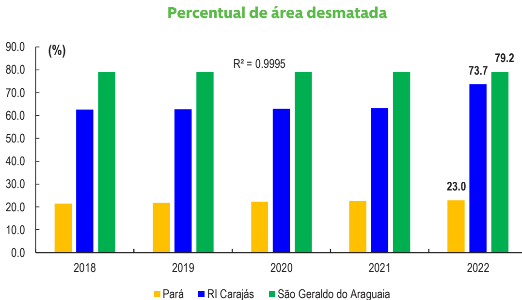
Gráfico 25: Percentual de área desmatada, Pará, Região de Integração Carajás e São Geraldo do Araguaia, 2018 a 2022
