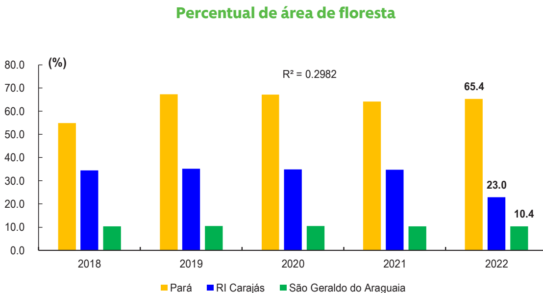
Gráfico 26: Percentual de área de floresta, Pará, Região de Integração Carajás e São Geraldo do Araguaia, 2018 a 2022.
